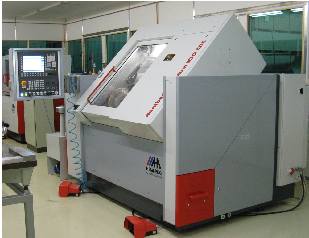
Hembrug Slantbed Mikrotorn 100 CNC high precision turning lathe / Hembrug Slantbed Mikrotorn 100 CNC nagy pontosságú eszterga Price: 152 000 EURO / Ár: 45 600 000 HUF
